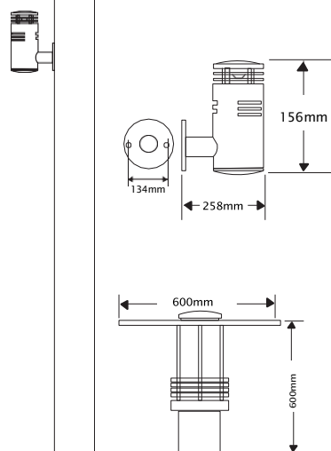
CLIMA WALL BRACKET FYZT-8021-WB
