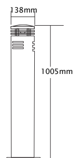
CLIMA BOLLARD FYZT-8021-B
